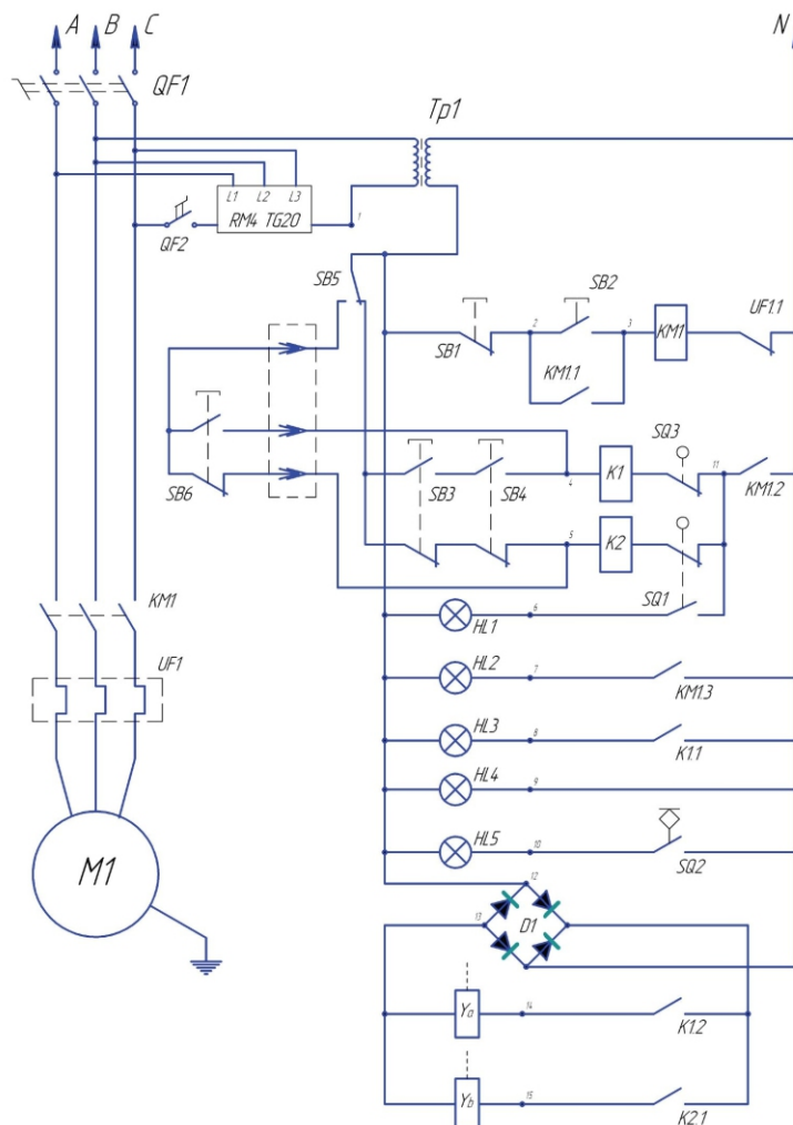
Рис. 4. Схема электрооборудования «Ажур-3М»
