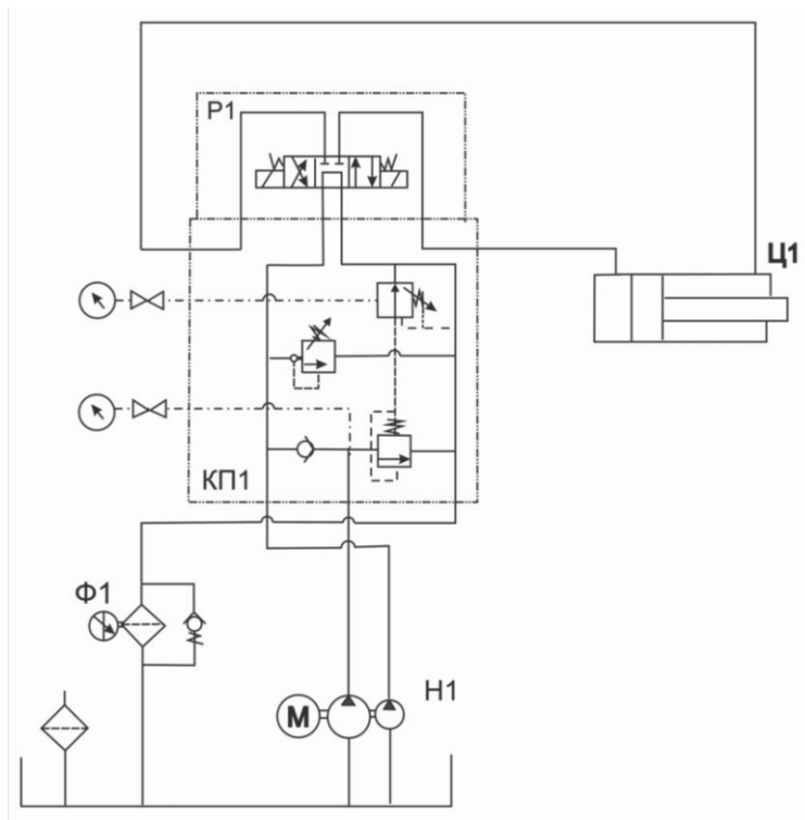
Рис.2. Гидравлическая схема пресса
