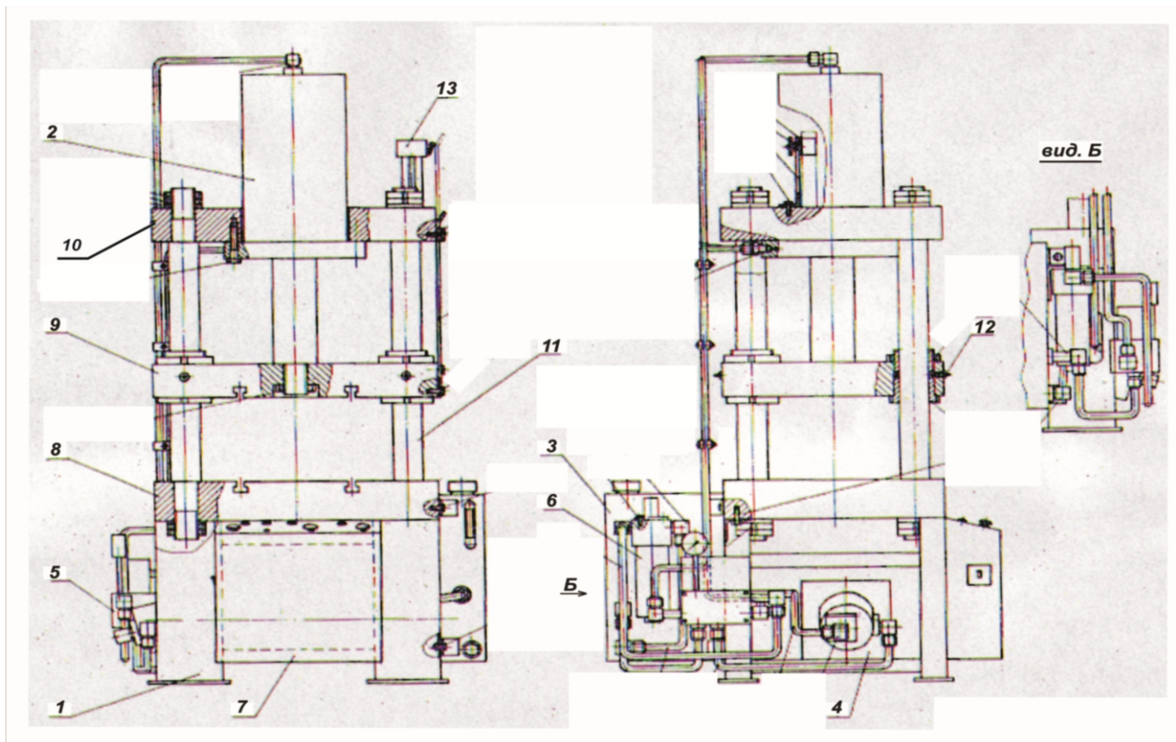
Рис.1. Пресс
